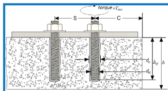
FIGURA 2 - Detalle de instalacion tipica para varilla roscaada o barra de construccion.
