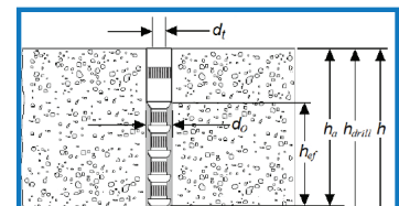
FIGURA 3 - Detalle de instalacion tipica para insertos internamente roscaados.
